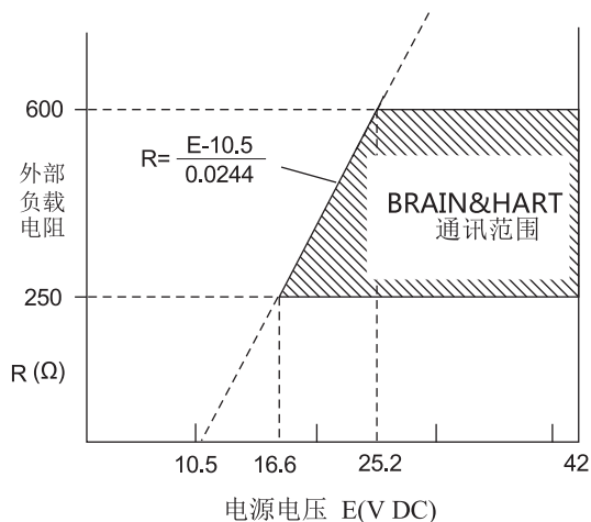
图 1： 电源电压与外部负载电阻之间的关系 （输出信号代码 D & J）
